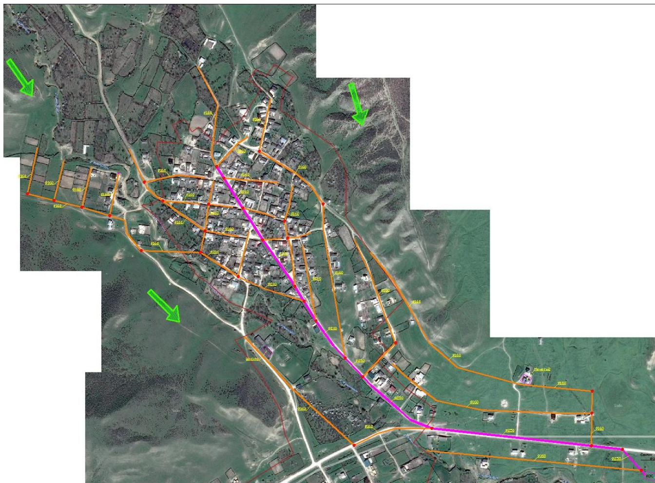
Рис 12.1. Схема водоотведения с. Джаванкент на перспективу
